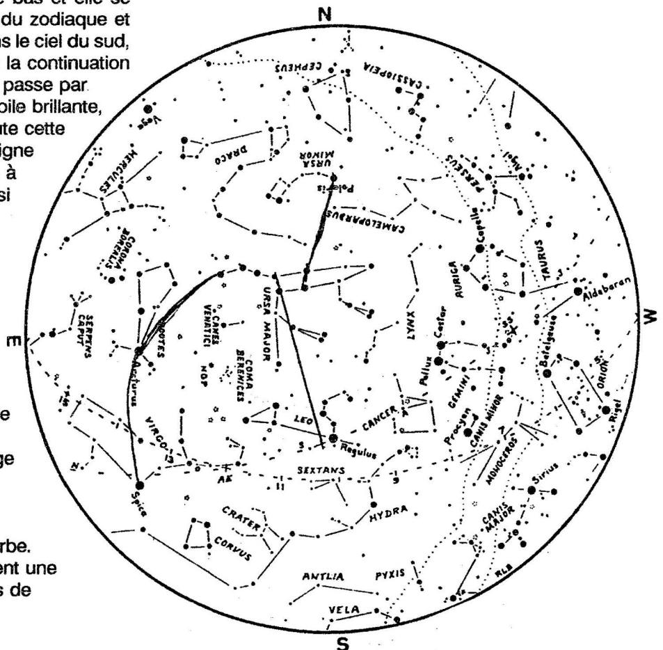
La carte du ciel
